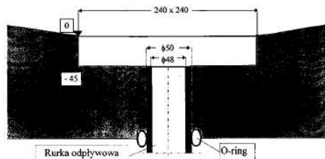
Rys. 6 Szcik sposobu osadzenia sączka - Wariant II - Etap I
